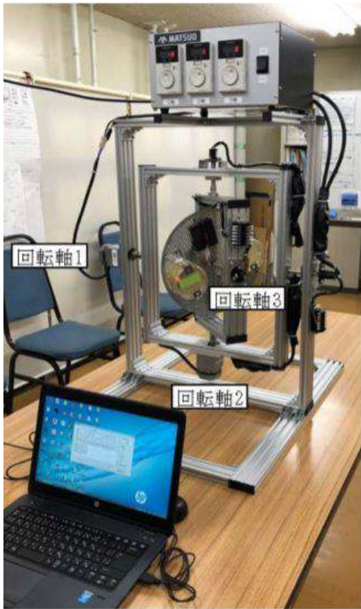
図1 開発した3軸クリノスタット
